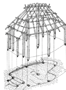
Schema di costruzione di una capanna in legno.
